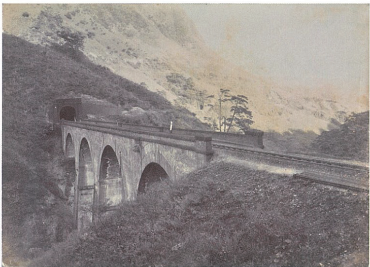
信越本線・碓氷第三橋梁 明治後期
